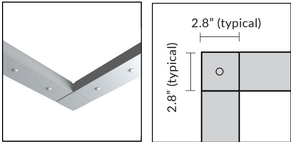
"L" Joiner MS-ACJL-BL MS-ACJL-WH
