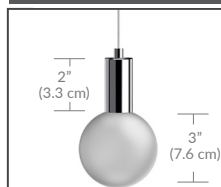
FROSTED ACRYLIC 3" GLOBE GLSFR
